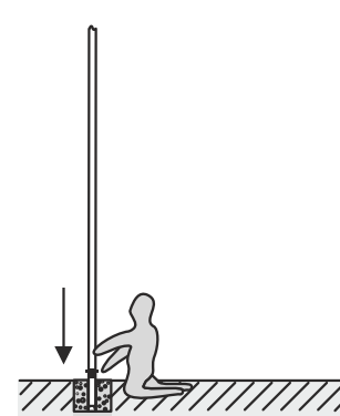
Zentrierung einstecken
